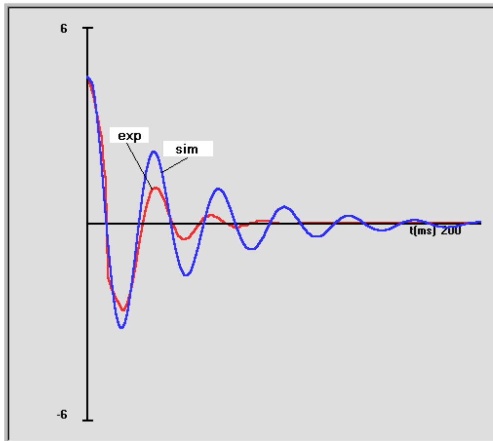
Fig 2.- Experimento y simulación de un circuito RLC
