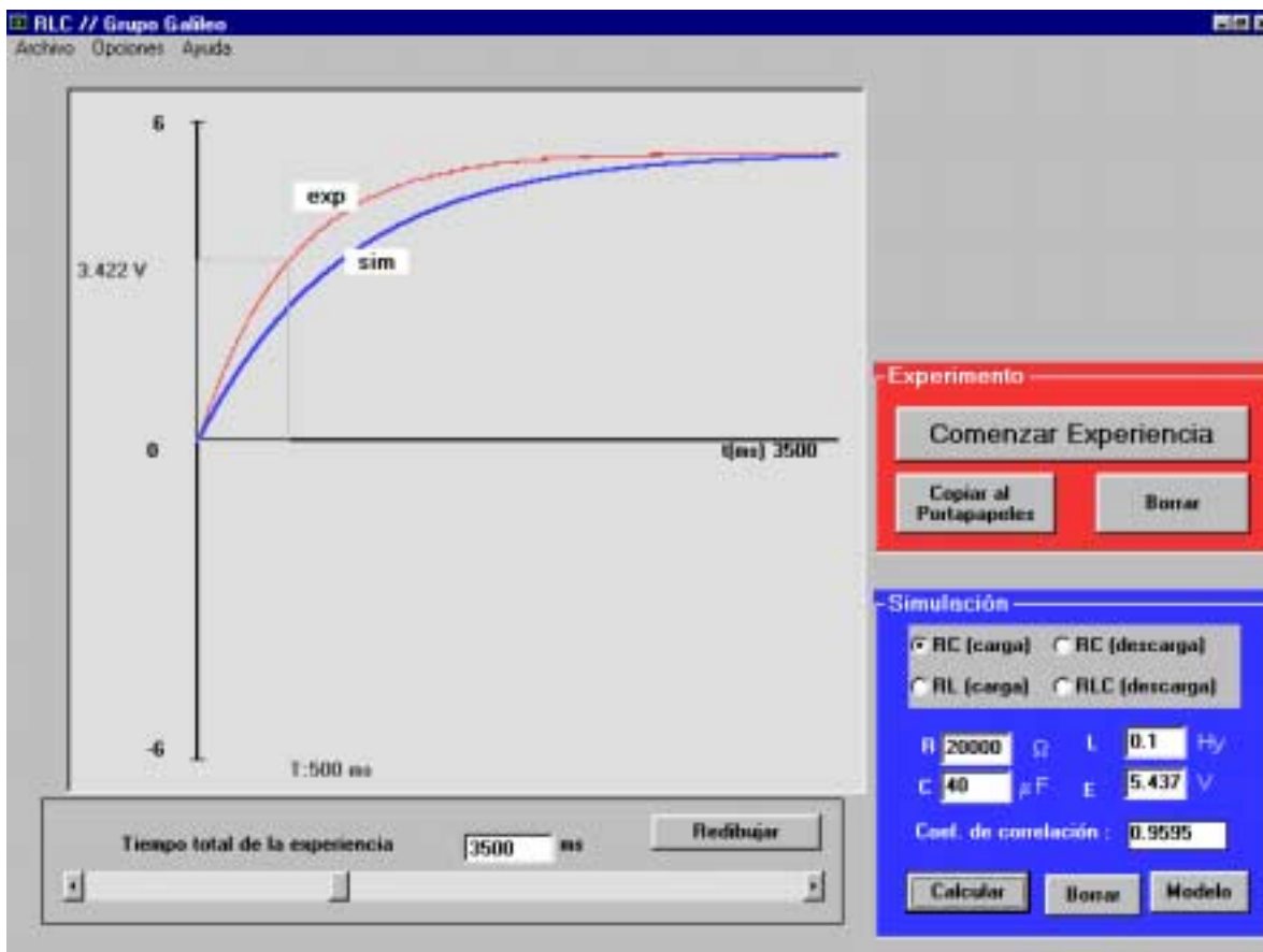
Fig 1.- Visualización de la gráfica experimental y una simulación para un circuito RC en carga
