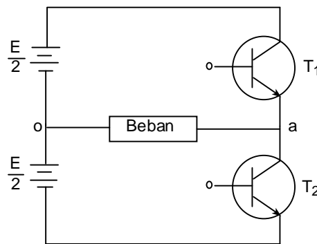
Gambar 2.1 Inverter satu fasa jembatan setengah
