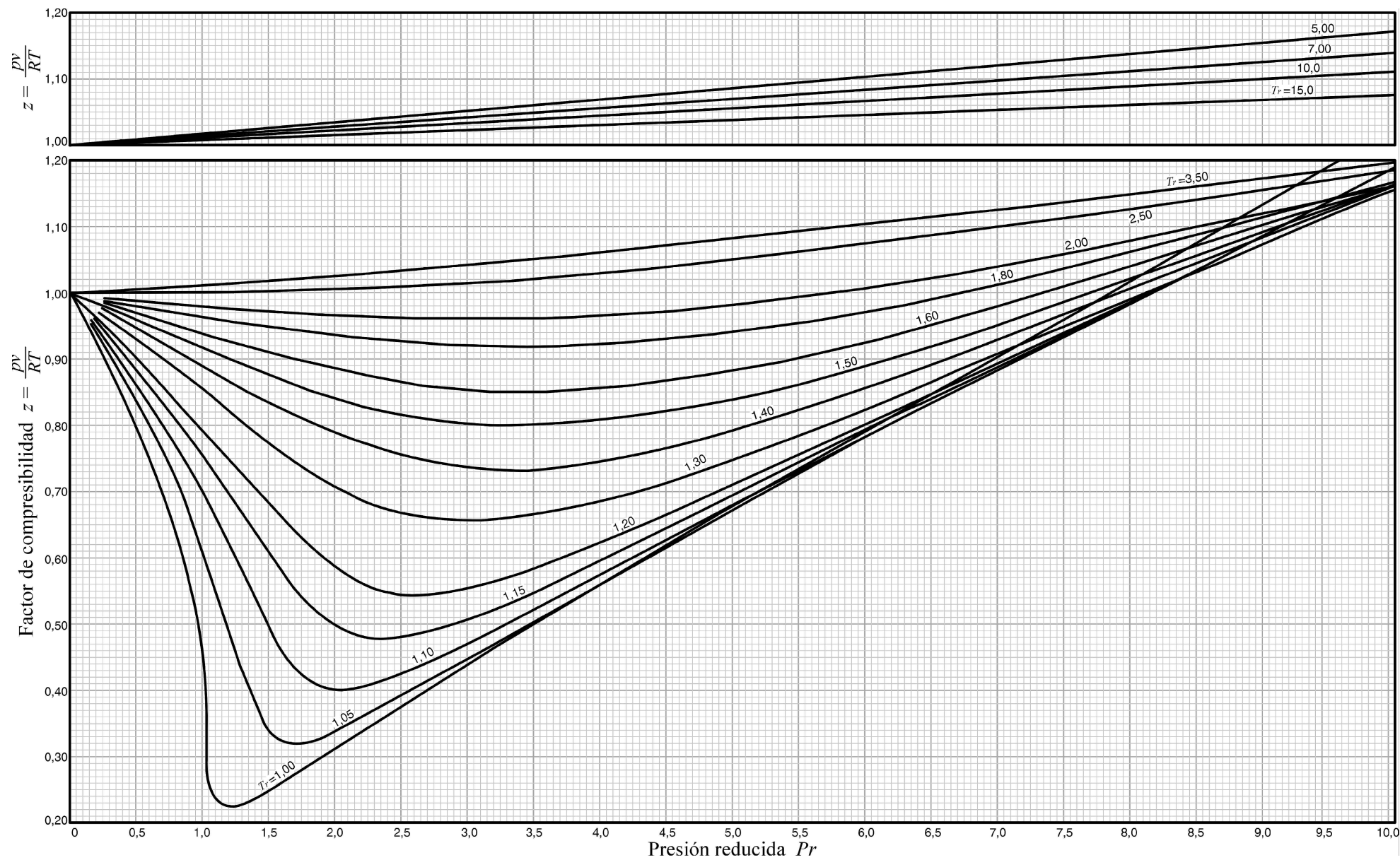
Diagrama de compresibilidad generalizado de Nelson-Obert (presiones medias).
