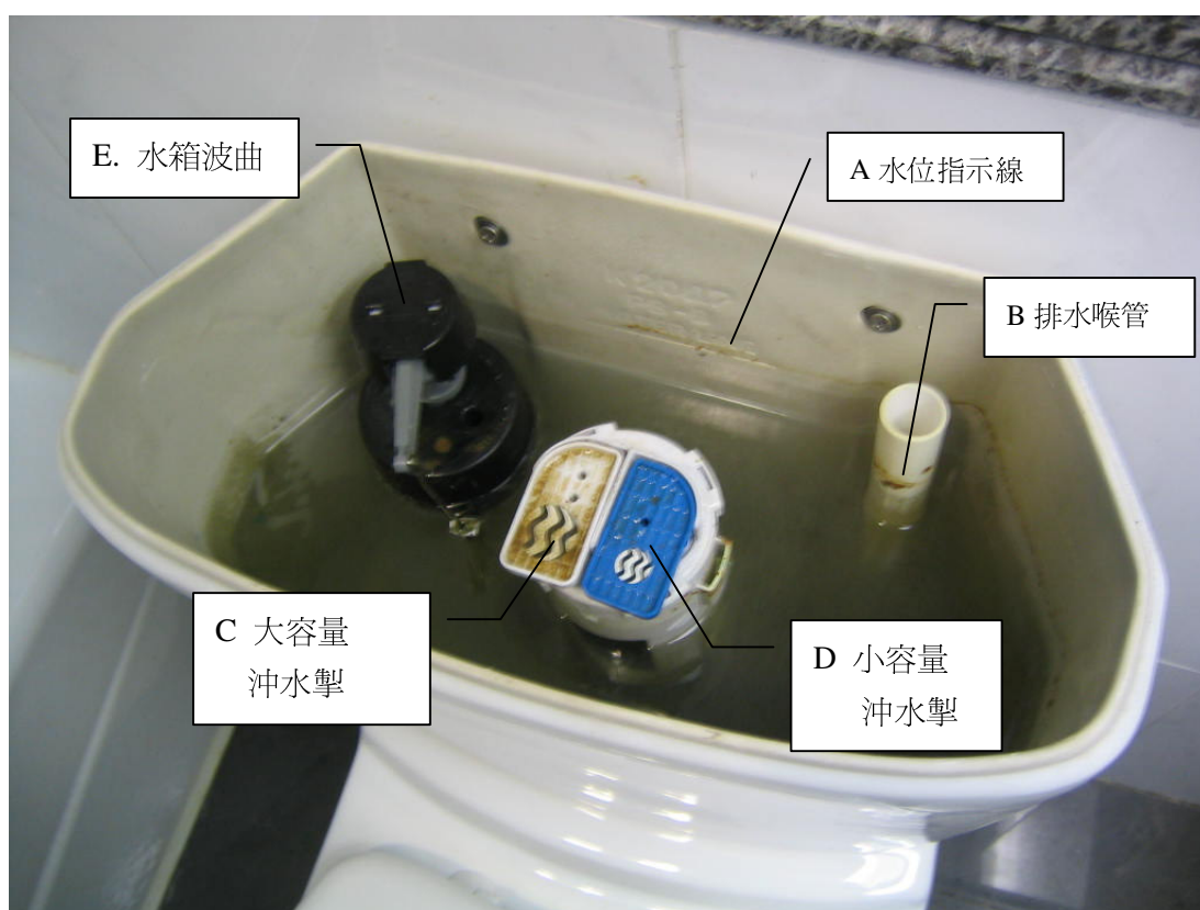
圖 12) 水箱內部位置圖
