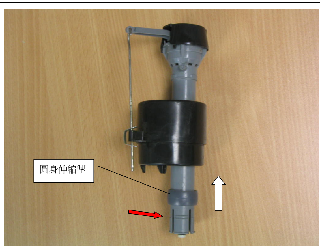
圖 5) 水箱波曲經其底部之膠軸(紅箭咀示)連接水箱。請向上提起圓身伸縮掣以拔起波曲。
