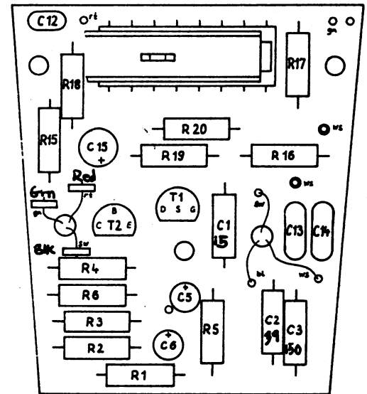
Bestückungsplan component locations
