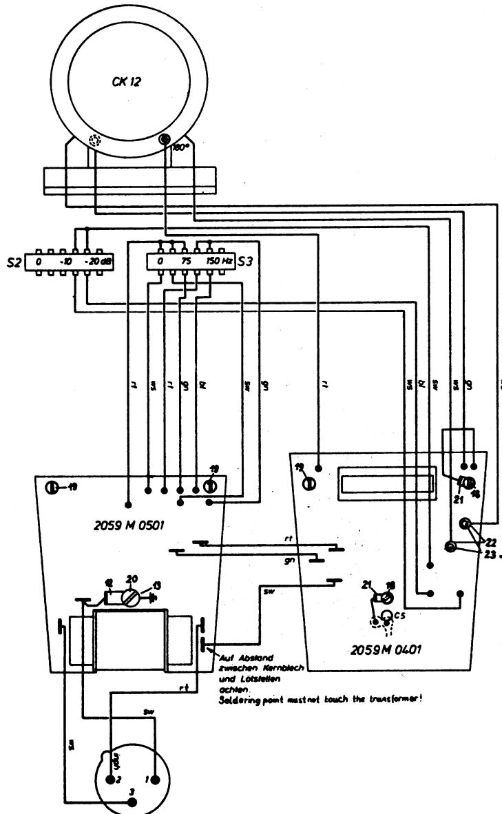
Verdrahtungsplan wiring diagram
