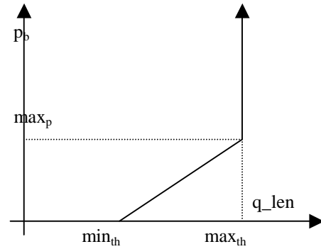
Figure 2. RED parameters
