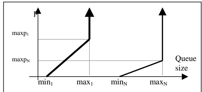
Figure 16. RIO parameters
