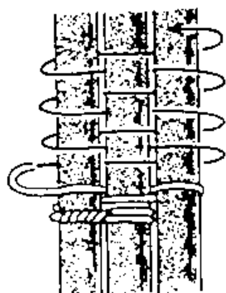
1 如圖所示，利用八字纏繞的方法來組合三腳架，是最適合不過
