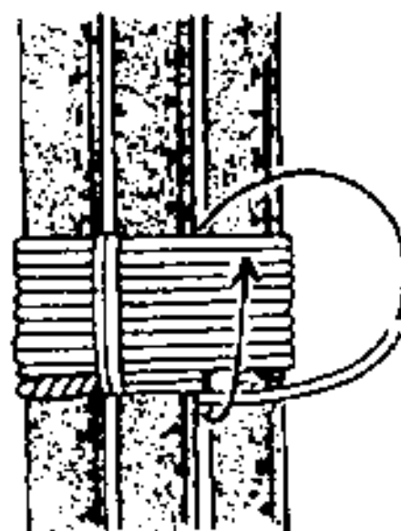
3 接著把繩索穿過圓木之間 3 圈左右
