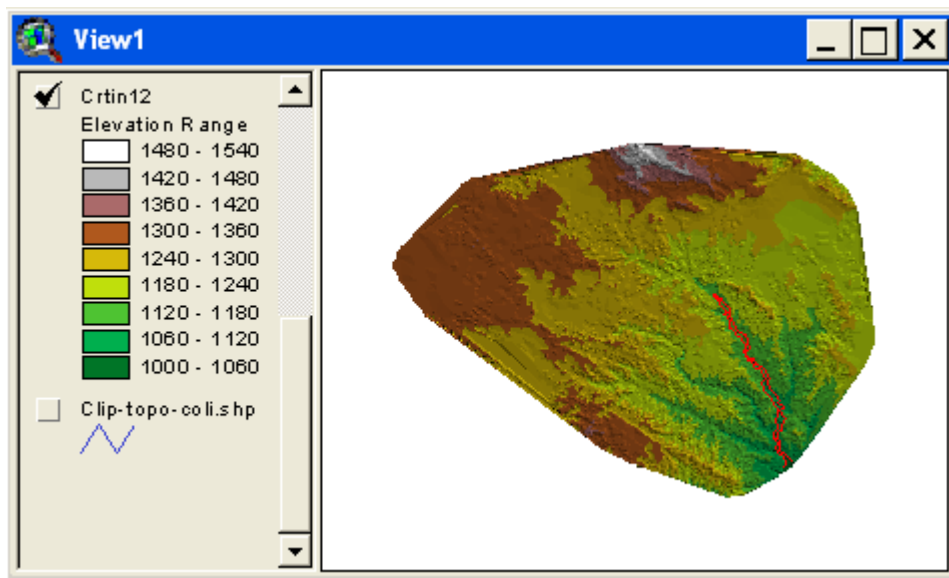
شکل (1) - TIN تهیه شده از سطح زمین
