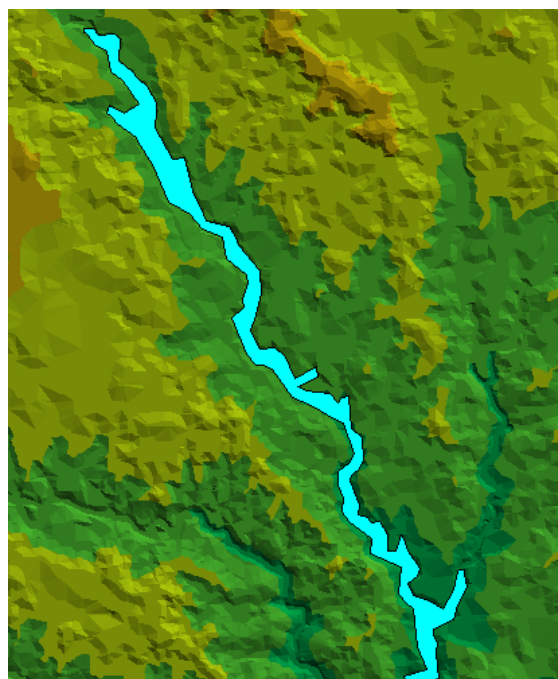
شکل (5) - پهنه بندی سیلاب 25 ساله بر روی TIN زمین
