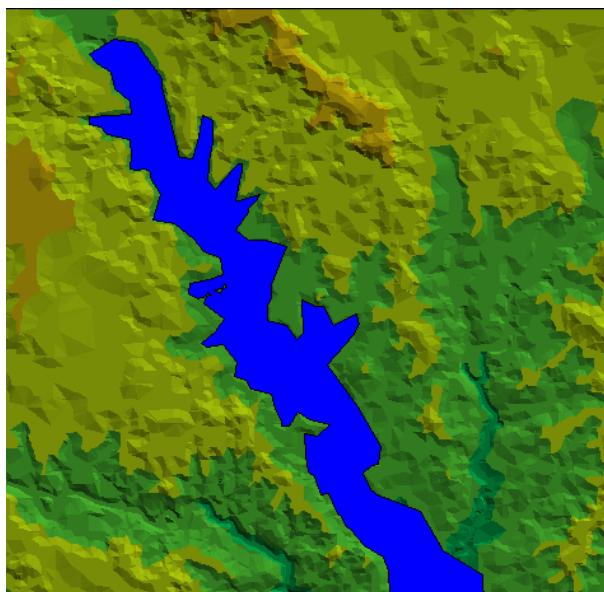
شکل (5)- پهنه بندی سیلاب 50 ساله بر روی TIN زمین
